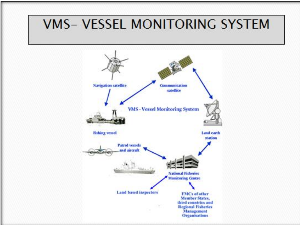
ကွန်ရက်ချိတ်ဆက် အလုပ်လုပ်ဆောင်ပုံ (ဌ-၂)
