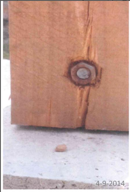
ကျောင်းဆောင်သစ်တွင် စံချိန်စံညွှန်းမမီသည့် ၆” x ၆” တိုင်များ စိုက်ထူထားပုံ (က-၁)
